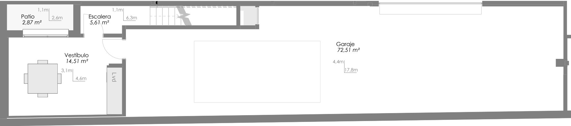
Planta sótano
