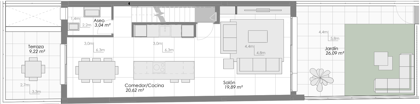
Planta sótano
